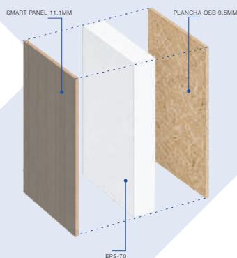
MUROS DE PANEL SMART SIP
